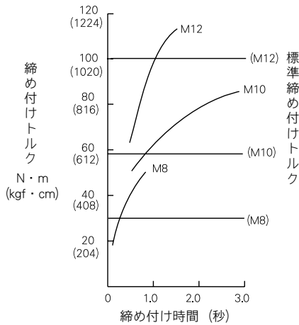
高力ボルト
