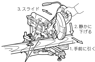
スライド軸固定用 ツマミネジ
