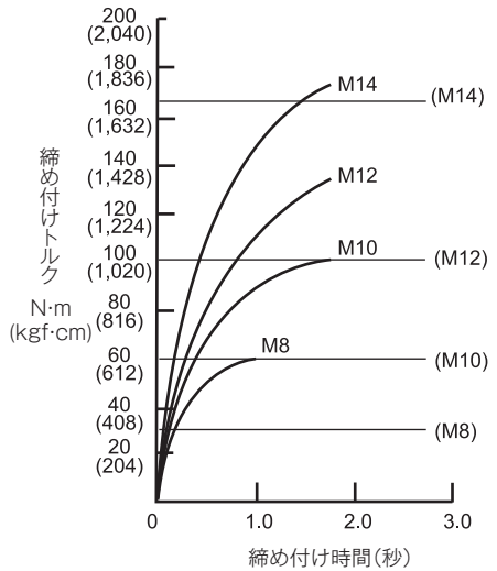
高力ボルト
