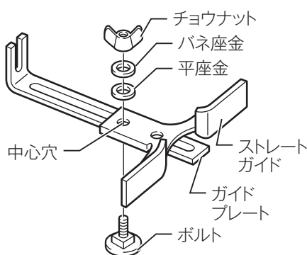
半径121~221ミリの円を加工する時
