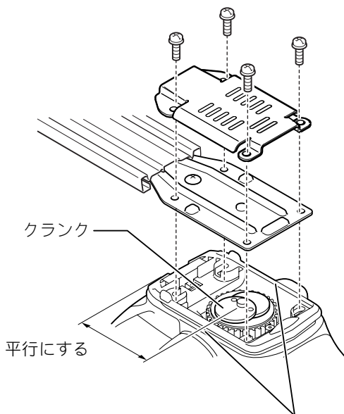
ハウジング部拡大図
